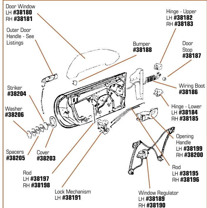
#38184 1997-2004 Door Hinge - Lower - LH
